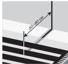
Рис. 1. Схема установки датчика температуры пола
