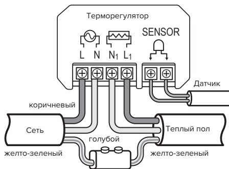
Подключение к 2-х проводной линии
