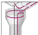
Монтаж кабеля на водосток
